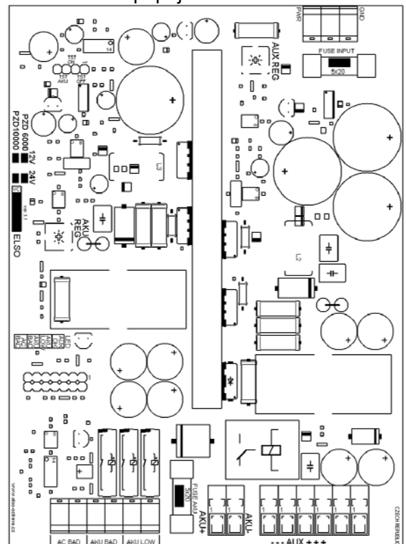
PZD10 připojení svorek
